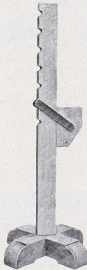
N° 206 SERVANTE POUR ÉTABLI
